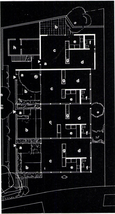
Grundriß der Häuser 1 bis 4 / Plan des maison 1—4 / Plan of houses 1—4
