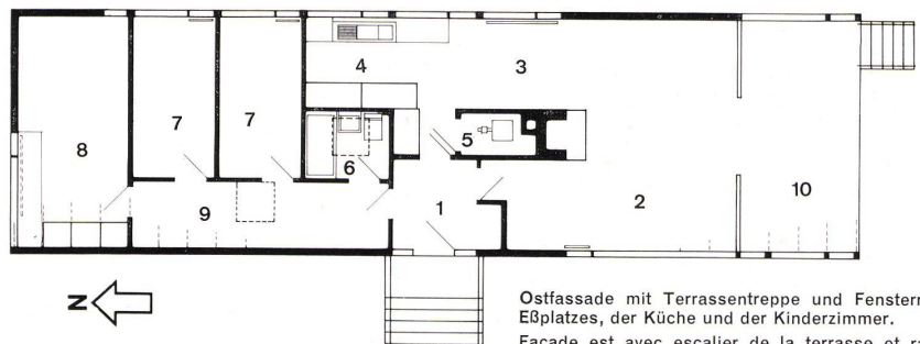
Erdeschoß Grundriß 1:150.
