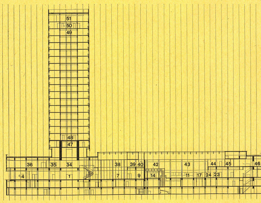
3 Schnitt AA 1:800. Coupe AA. Section AA.
