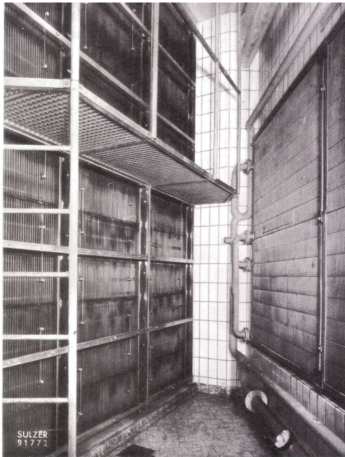
Ausschnitt aus der Frischluft-Aufbereitungszentrale
