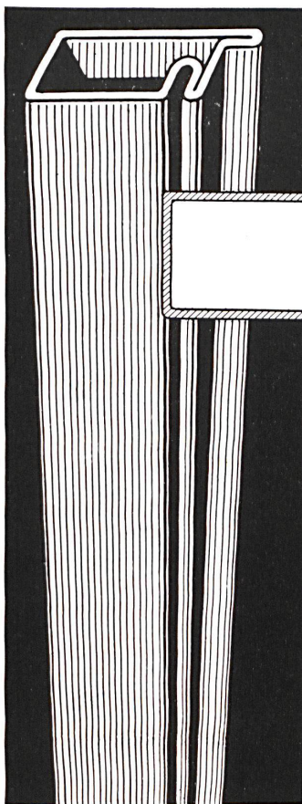
Kittleiste aus Hart-PVC Dichtung aus Kunststoff
