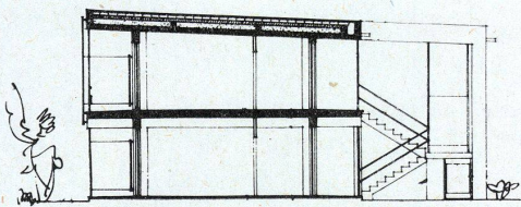
C Schnitt durch Zimmer 1:250. Coupe de la chambre. Section of room.
