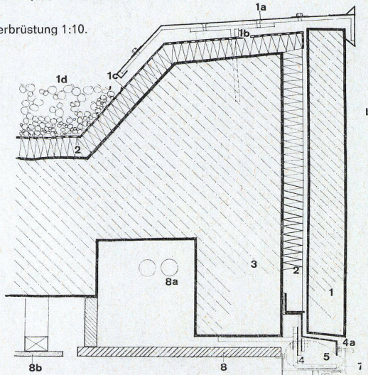
Detail VII: Plattenaufhängung / Suspension des plaques / Slab hanging
