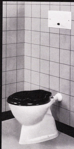
GEBERIT-PVC-Spülkasten für Wandebau Nr. 15.000, mit Spülrohranschlussgarnitur Nr. 44.212 für am Boden befestigtes Klosett
