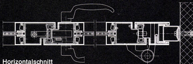
Horizontalschnitt
