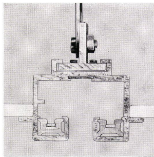
Aufhängen in Verbindung mit Deckenplatten
