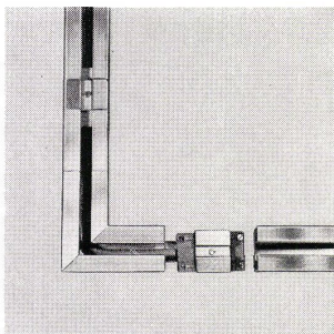
Verbinden mit Eckstück und einschiebbarem Kontaktapparat
