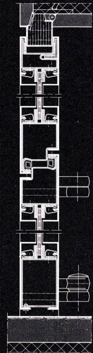
Vertikalschnitt
