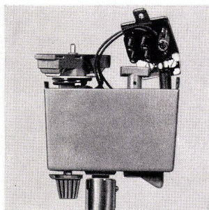
Anschliessen der Leuchte am Adapter
