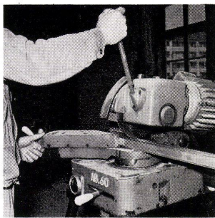
Ablängen der 5 m Schienen auf der Baustelle
