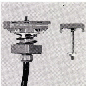
Stromabnehmer und Befestigungsbolzen für Fluoreszenz-Leuchten
