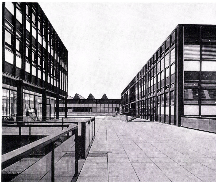
1 Gesamtanlage mit Freilufttribüne, Leichtathletikhalle, Forum und Zentralbau.
