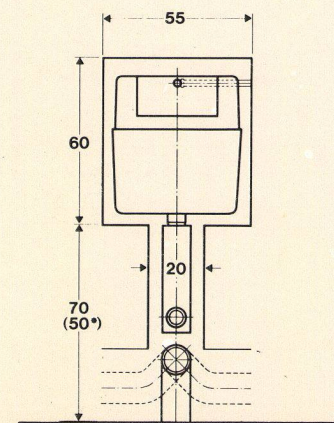
Aussparungsmasse
