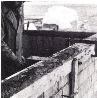
9 Zementmörtel einfüllen Remplir de mortier
