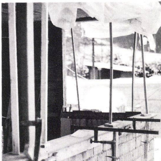
13 Versprüssen Étayer
