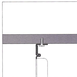
17 Anschrauben oder kleben Visser ou coller
