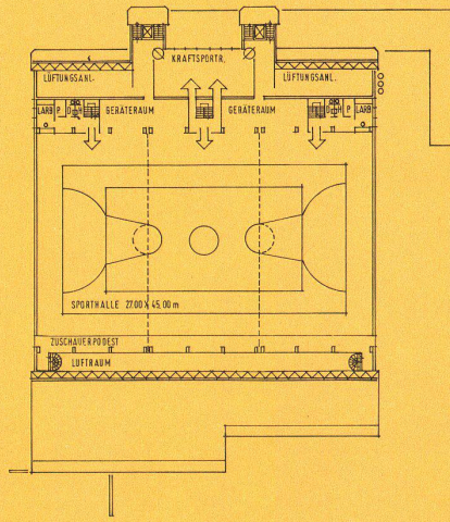
ERDGESCHOSS
