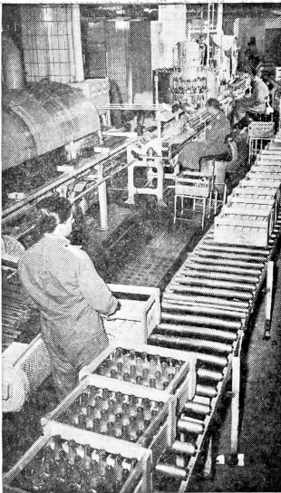
Teilansicht des Maschinensaaus von der Waschmaschine bis zur Korkmaschine.
