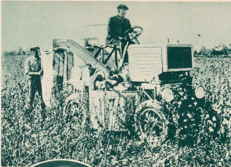
Die Baumwollentemaschine.
