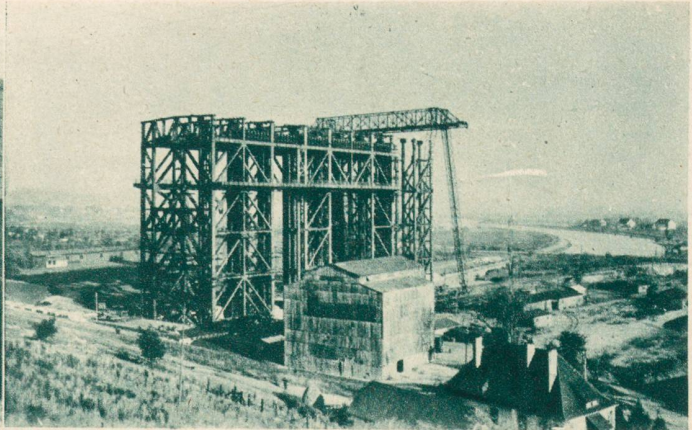
Ein riesiges Schiffshebewerk in Niederfinow (Deutschland), um Schiffe von einem Kanal in einen höher gelegenen zu heben. Atlantic-Photo.
