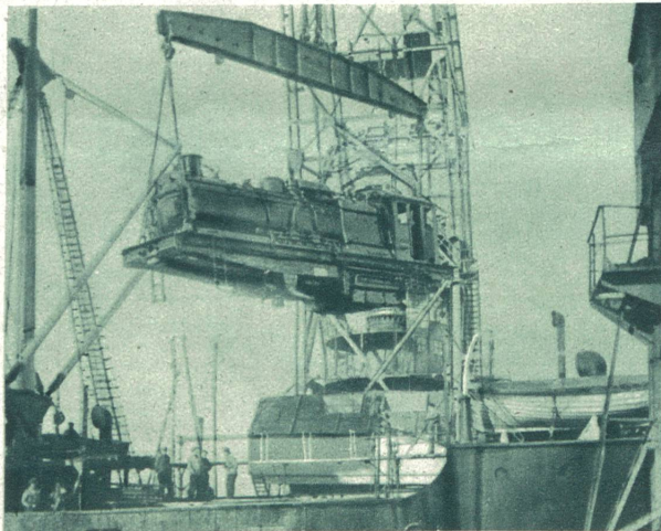
Im Hafen von Dünkirchen (Frankreich, am Kanal). Mit spielender Leichtigkeit hebt der schwimmende Kran die Schnellzugslokomotive auf den Frachtdampfer.
