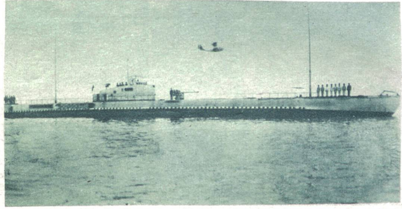
Das französische Unterseeboot »Prométhée« sinkt mit 65 Mann. Auf der Höhe von Cherbourg ist das Unterseeboot, wie jetzt festgestellt werden konnte, unter Wasser auf einen Fels aufgefahren. Photo Keystone.
