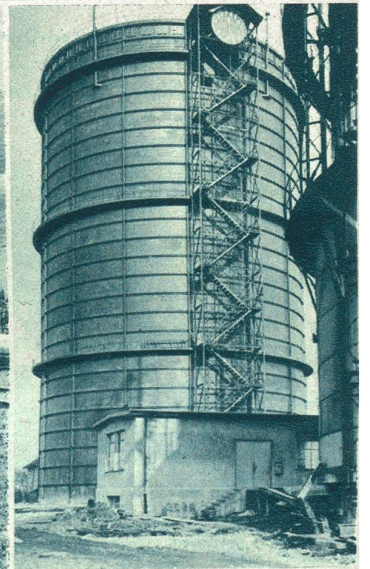
Der neuerbaute Gaskessel der Stadt Biel, einer der größten Kessel dieser Art in der Schweiz (Höhe 38 Meter). Die Anlage wird demnächst in Betrieb genommen. Phot. W. Schweizer, Bern.
