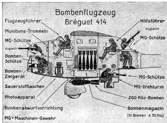
Querschnitt durch das Bombenflugzeug Bréguet 414.
