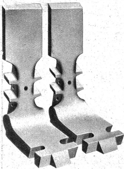
ZENT- Einsatzrost Holz- und Torf-Feuerung
