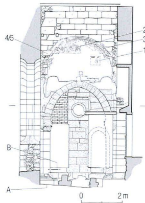
Mur est/Ostmauer
