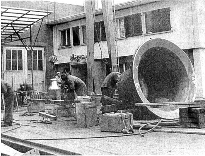
Abb. 3: Die g° Glocke für Kreuzlingen liegt 1964 für die abschliessenden Putz- und Polierarbeiten im Hof der Gieserei Eschmann in Rickenbach. / La cloche en sol2 destinée à Kreuzlingen, finitions dans la cour de la fonderie Eschmann à Rickenbach en 1964. (Foto Nachlass Emil Eschmann)
