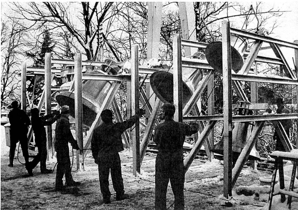
Abb. 5: Das gis°-Geläute von 1968/69 für die neu erbaute Pfarrkirche St. Gallus in Lichtensteig wird in Rickenbach zur Probe geläutet. / Sonnerie en sol#2 de 1968/69, destinée à la nouvelle église paroissiale de St-Gallus à Lichtensteig, sur le banc d'essai à Rickenbach. (Foto Nachlass Emil Eschmann)
