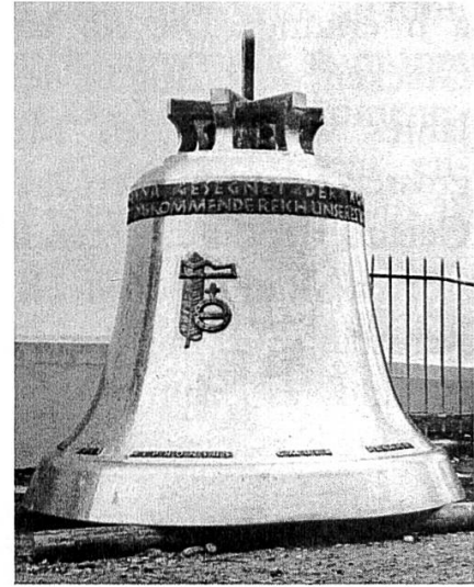
Abb. 4: Die fertige g°-Glocke für die Basilika St. Ulrich & Afra in Kreuzlingen. Mit 6'285 kg handelt es sich um die grösste von Emil Eschmann gegossene Glocke. / La même cloche terminée. Avec ses 6'285 kg, il s'agit du plus grand bourdon fondu par E. Eschmann. (Foto Nachlass Emil Eschmann)
