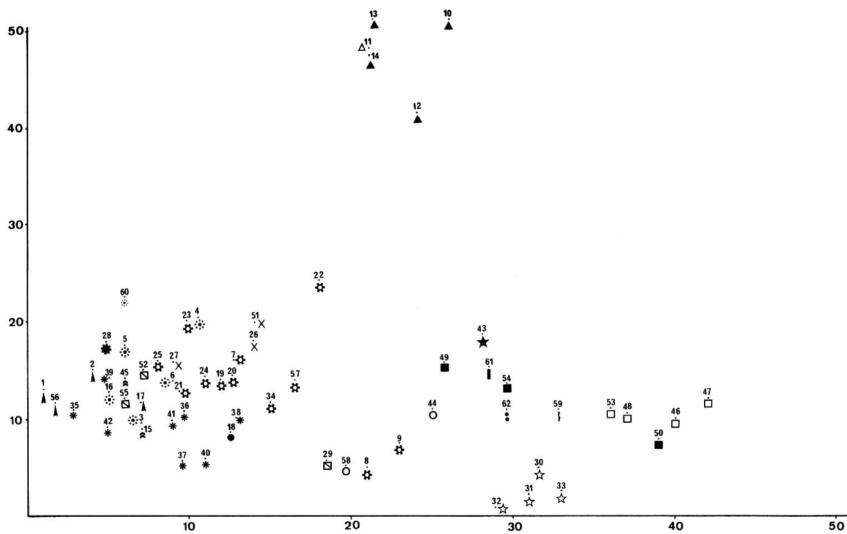
Fig. 3. — Representación de eigenvectores (ejes 2 × 3).
