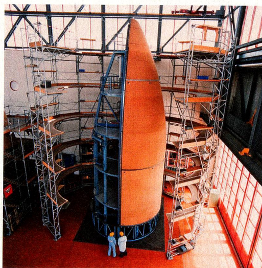
Construction de missiles à Emmen, 1992
