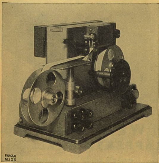
Registrier-Chronograph Typ M 427
