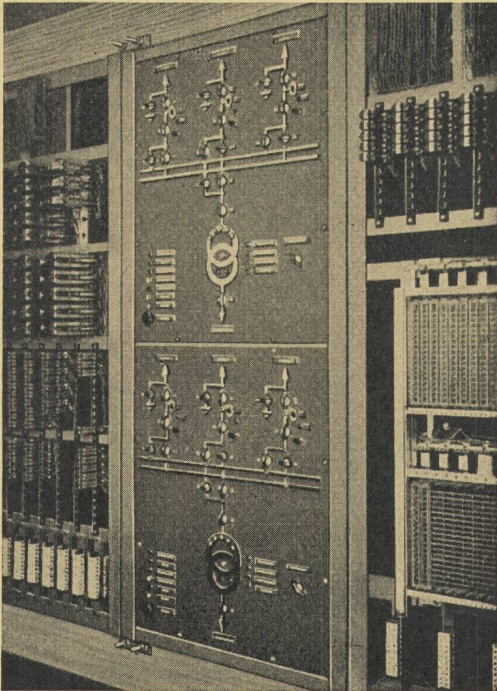
Fernsteuerungsanlage mit Verwendung von Kombinationsrelais und Kreuzwählern
