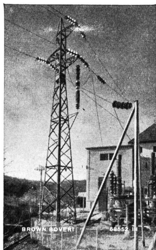
Fig. 3. HF-Telephonieverbindung Montcherand-La Peuffaire über die 125-kV-Hochspannungsleitung mit am Mast aufgehängtem Kopplungskondensator und Doppelwellensperre
