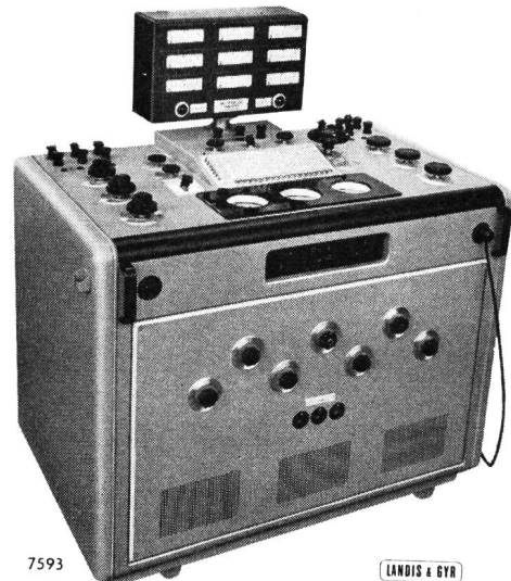
Fig. 6. Eichstation «Metrabloc» für Elektrizitätszähler
