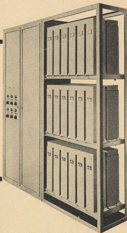
Automatische Blindstromkompensationsanlage, Blindleistung 240 kVar, Spannung 380 V s
