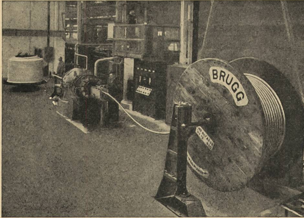
«Kontinuierliche Bleikabelpresse»
