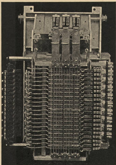
Kreuzwähler
