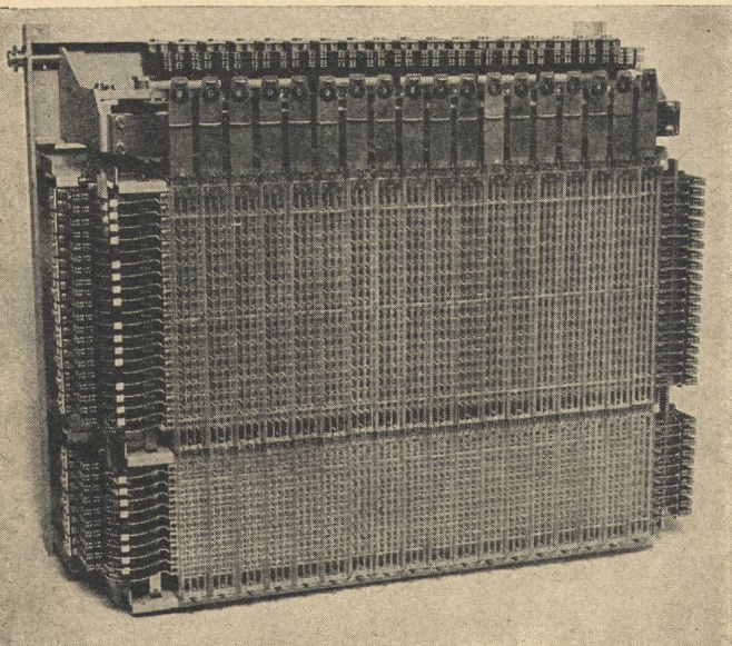
Kreuzwähler K 53
