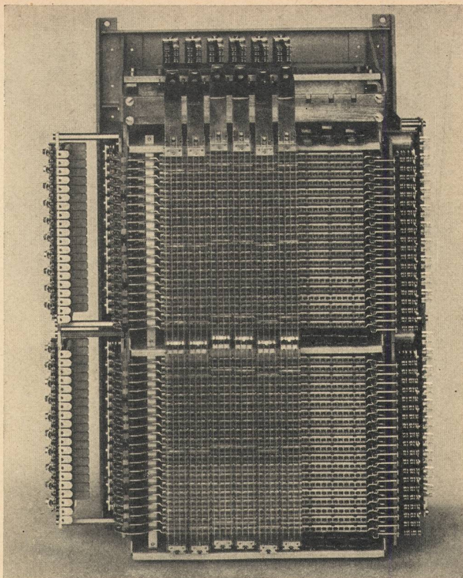
Kreuzwähler K 53
