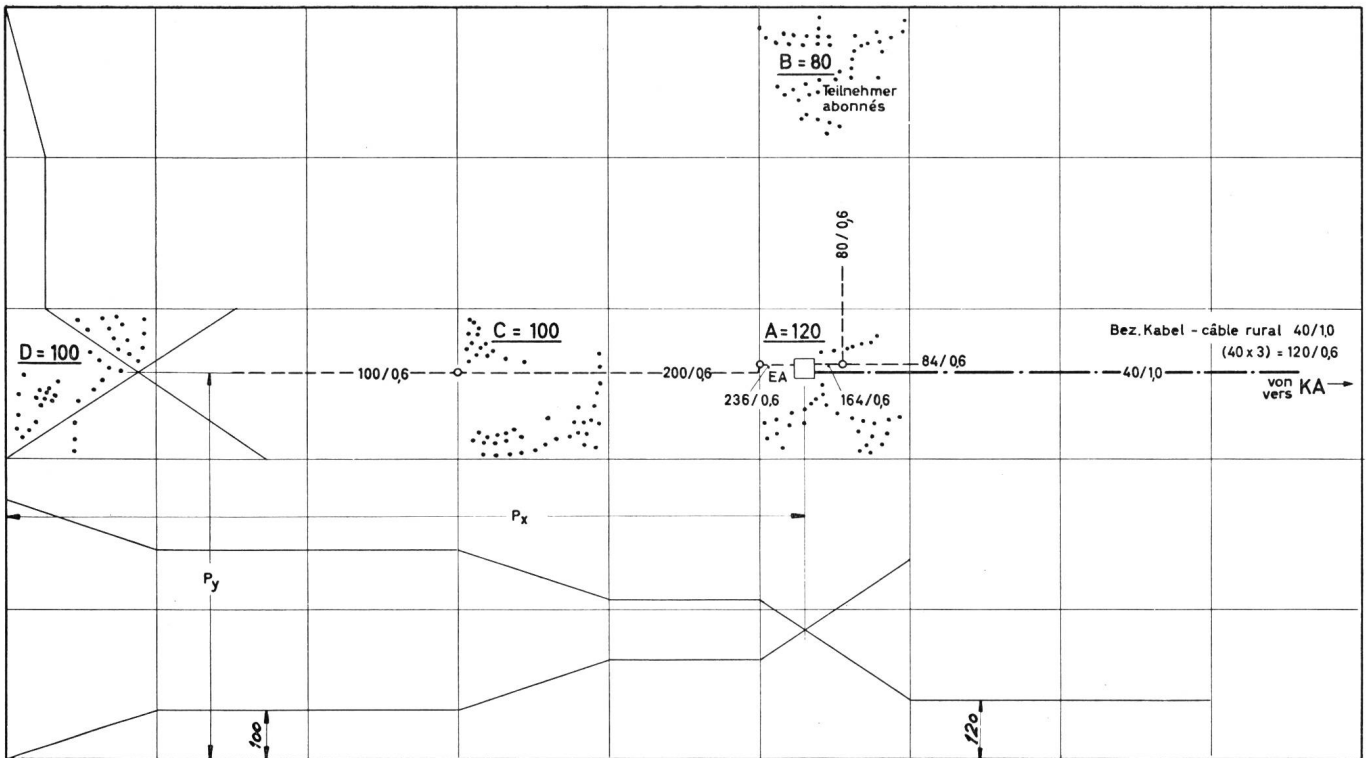
Fig. 4. Arithmetische Methode zur Bestimmung des Netzschwerpunktes Méthode arithmétique pour la détermination du centre de gravité du réseau téléphonique
