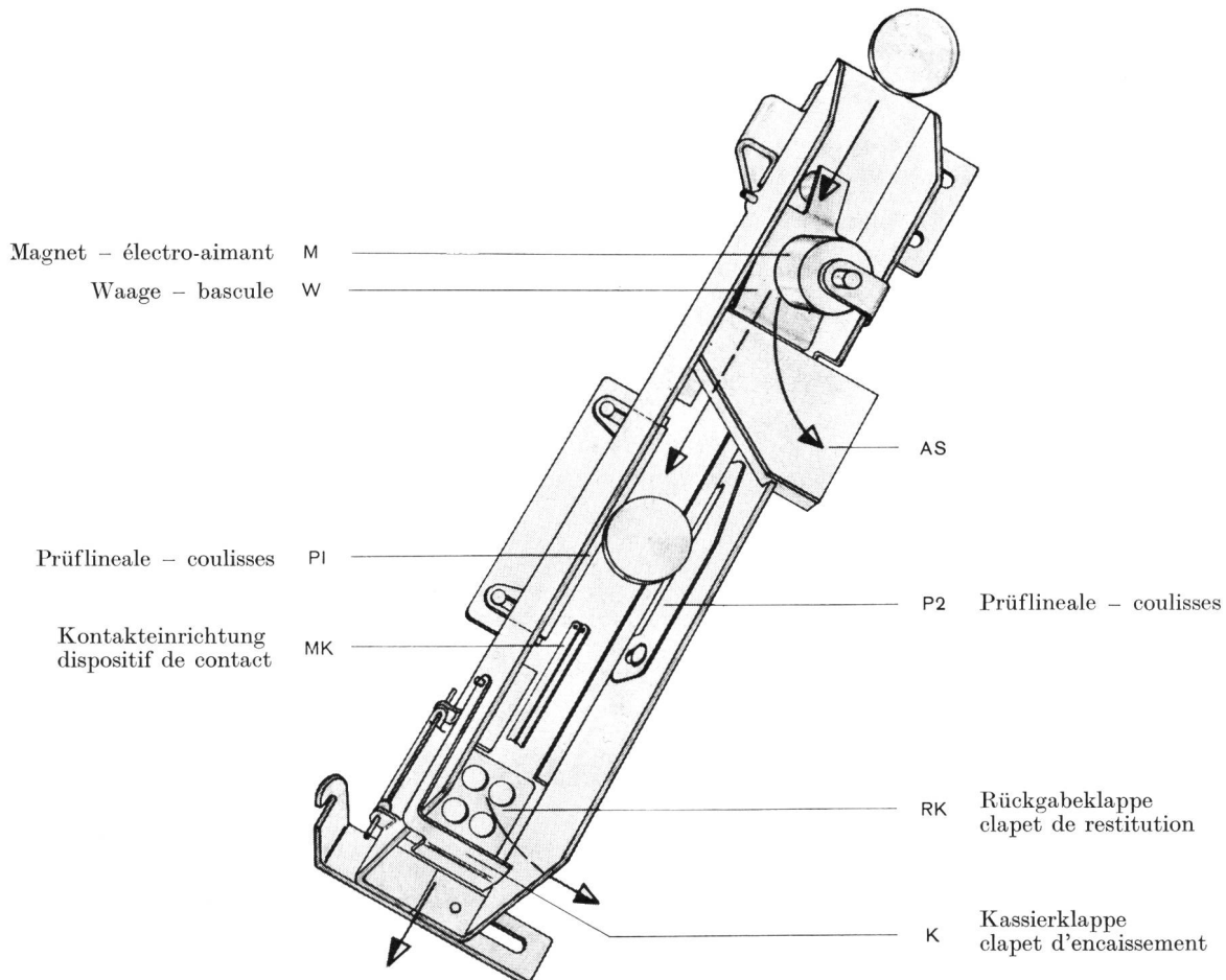
Fig. 4. Funktionszeichnung Münzkanal – Fonctions du canal de monnaie
