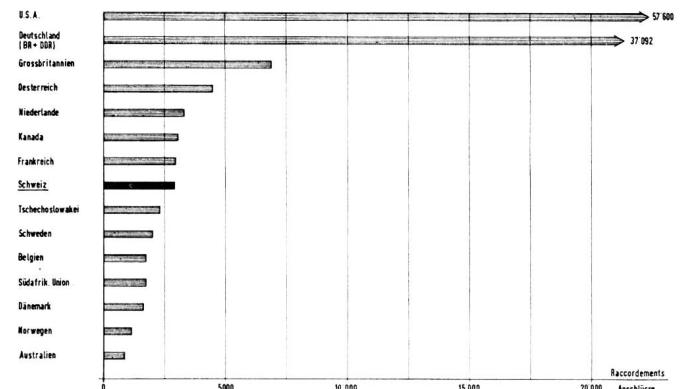
Fig. 2. Zahl der Telex-Anschlüsse am 1. Januar 1961 Nombre des raccordements télex au 1 er janvier 1961
