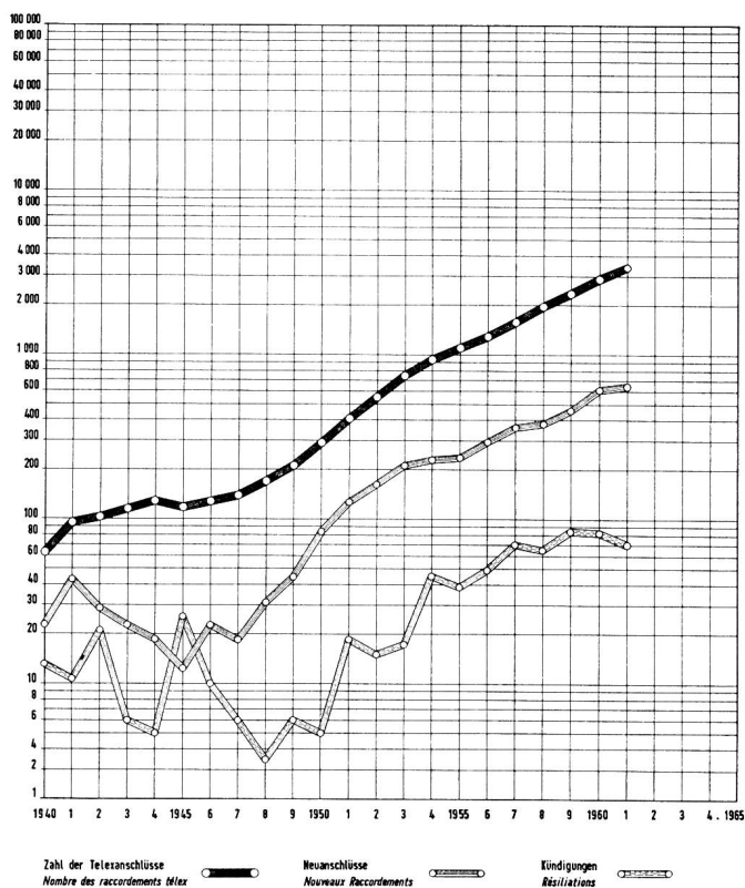
Fig. 4. Entwicklung der Zahl der Telex-Anschlüsse der Schweiz Développement du nombre des raccordements télex en Suisse
