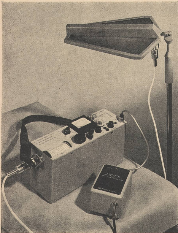
Feldstärke-Zeiger HUZE mit Messantenne und Ladegerät
