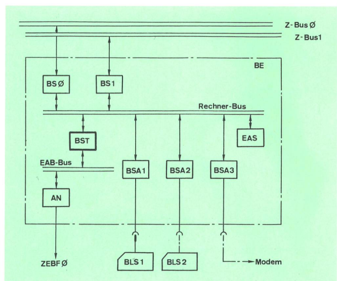
Fig. 6 Unité d'exploitation A 52 S/HS 52 B AN Circuit de connexion BST Commande de l'unité d'exploitation EAB-Bus Bus des modules entrée/sortie ZEBF Panneau de service de l'unité centralisée Z-Bus Bus centralisé (Autres abréviations voir le texte) Rechner-Bus — Bus de calculateur
