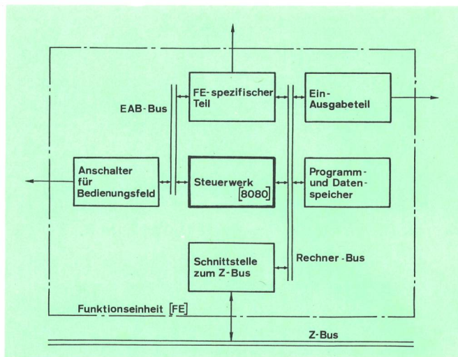
Fig. 2 Structure de principe d'une unité de fonction
