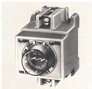
Parafoudre pour installations basse tension
