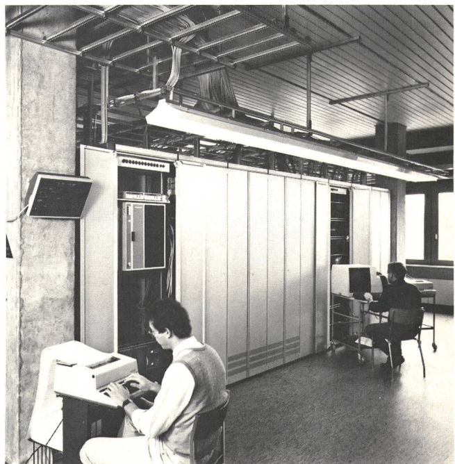
Fig. 5 Koordinationsprozessor CP mit Rechner SSP103D der Transitzentrale Bern-Ittigen – Processeur de coordination CP avec calculateur SSP103D au central de transit de Berne-Ittigen
