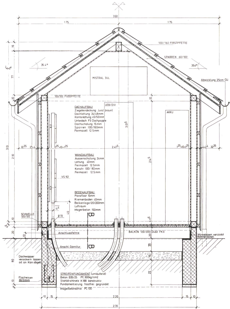
Bild 3. Querschnitt durch die Anlage.
