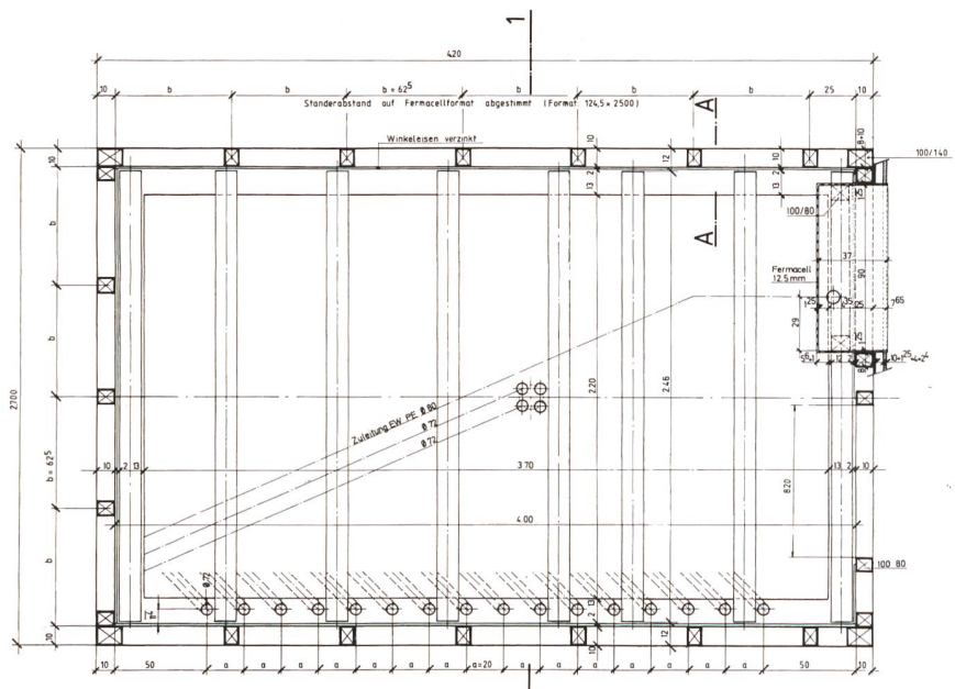
Bild 4. Grundriss.
