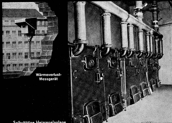
Selbsttätige Heizregelanlage
