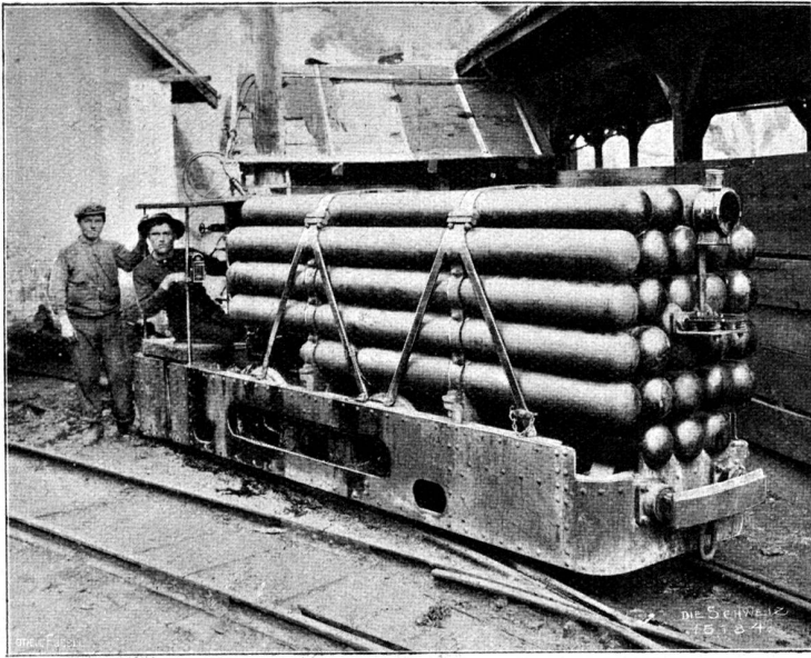
Die Tunnellokomotive, mittelst komprimierter Luft zu betreiben.
