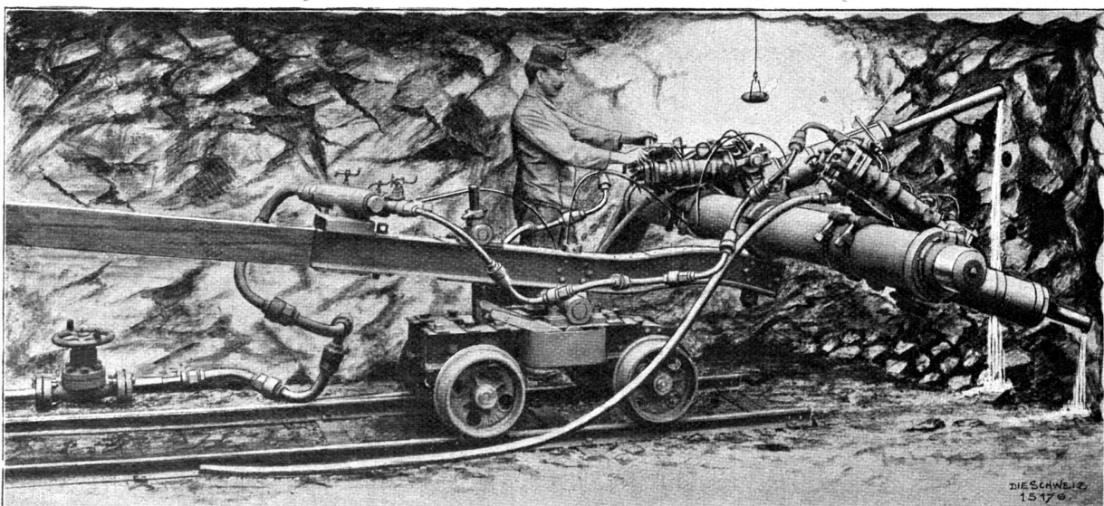
Die Brandtsche Gesteinbohrmaschine.
