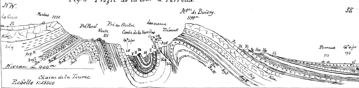
Fig. 3 Profil de la Cour à Perreux.
