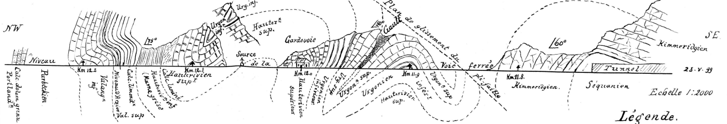
Fig. 2 Profil de la Tablette à Boudry.
