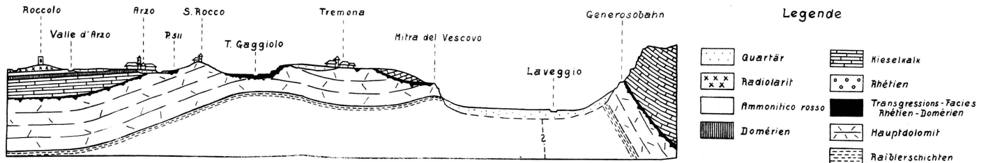
Sedimentationsverhältnisse des Lias am Alpenrand zwischen Mendrisio und Varese (schematisches Profil).
