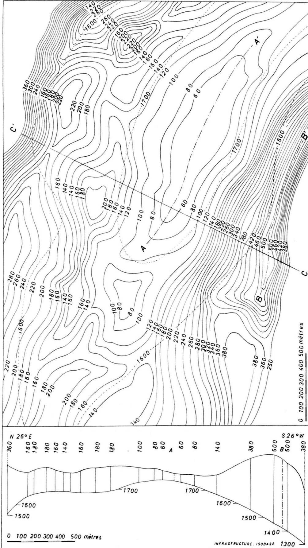
Fig. 2. Carte montrant un type de répartition des formations plastiques tel qu'il se présente dans de nombreux cas de disharmonie de plissement. — Isopaques des formations plastiques; AA' et BB', axes correspondant respectivement au minimum et au maximum d'épaisseur, 250 m. étant la moyenne en région non disloquée. - - - - - Isobases de l'infrastructure.
