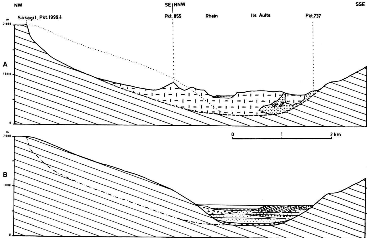
Fig. 3. Zwei Querprofile durch das Rheintal bei Tamins vor (B) und nach (A) dem Bergsturz aus dem Gebiet westlich des Kunkelspasses (Säsaig). Die Gleitbahn des Bergsturzes (strichpunktiierte Linie in Profil B) greift tief unter die Oberfläche der Talfüllung. Beim Abgleiten der Sturzmasse wird die Talfüllung durch die Bergsturzmasse seitlich weggeschoben, grossenteils verdrängt und ausgepresst (Profil A). Schief schraffiert: anstehender Fels. Mit der Schraffur ist zugleich die Schichtneigung angedeutet. Die Talfüllung in Profil B besteht aus Wasser, Seebodenlehm, Silten, Sanden, Schottern, Moränen und Bergsturzmaterial. In Profil A wurde die dünne Moränendecke auf dem Bergsturzmaterial weggelassen. Talfüllung und Bergsturzmaterial sind in beiden Profilen schematisch dargestellt.
