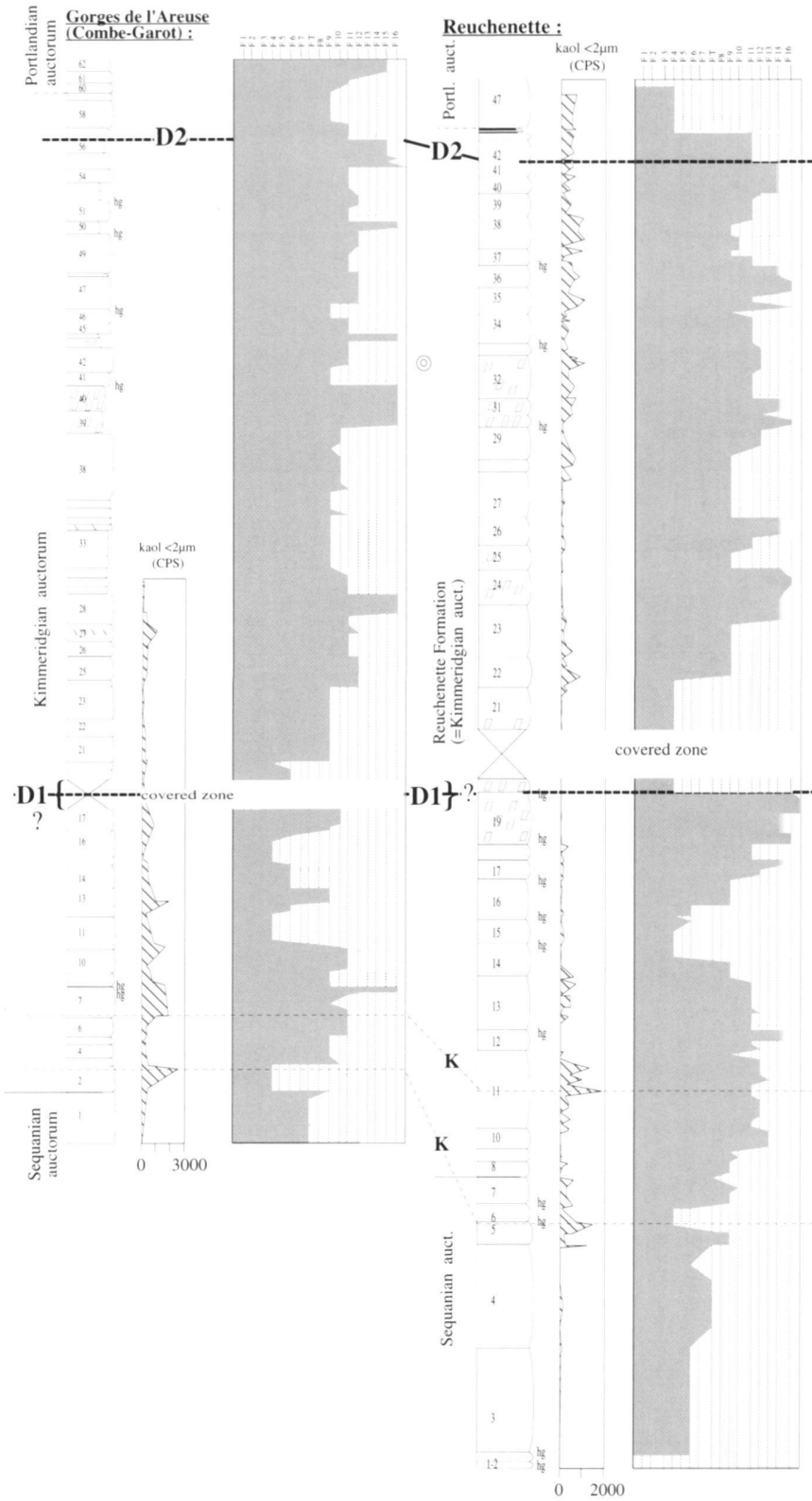
Fig. 10. Correlations based on microfacies evolution and kaolinite distribution (fraction <math>< 2\mu\text{m}</math>) at Morillon, Gorges de la Loue (A = Calcaires de Besançon, B = Calcaires et Marnes de Chargey, C = Calcaires à stromatoporiés de Matafelon, D = Calcaires des Fins, E = Calcaires de la Loue, F = Tidalites d'Arcsous-Cicon, G = Calcaires et Marnes de Savoyeux), Gorges de l'Areuse (Combe-Garot), Reuchenette and Vabenau. (bar = 10 m).
