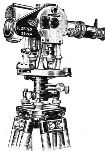
Reduktions-Tachymeter
