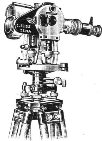
Reduktions-Tachymeter
